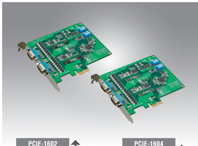
PCIE-1602
